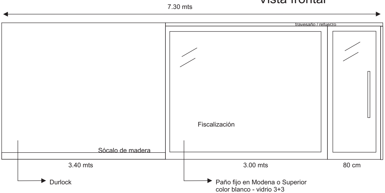
Fig. 2 - DIVISORIO DE DURLOCK y ALUMINIO (PERPENDICULAR A DIVISORIO DE DURLOCK)
