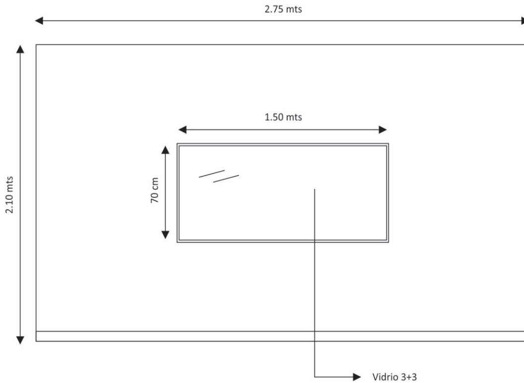
Fig. 1 - DIVISORIO DE DURLOCK (PERPENDICULAR A PARED DE MAMPOSTERÍA)
