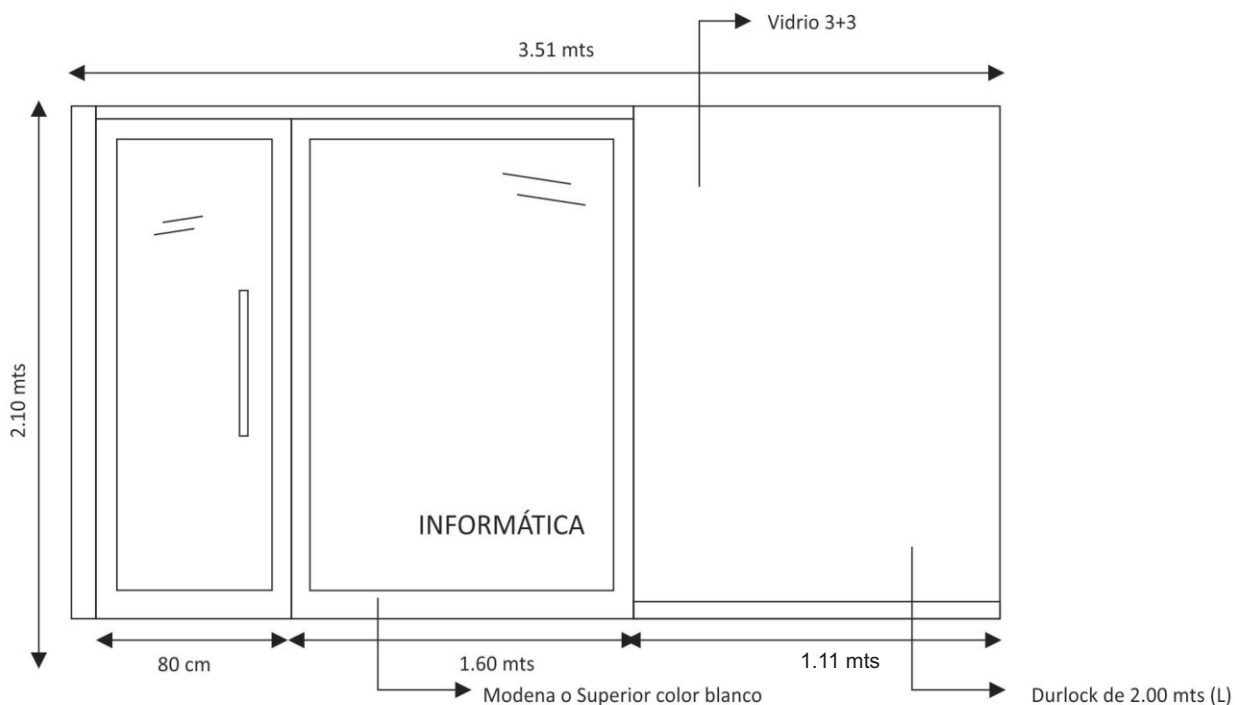
Fig. 2 - DIVISORIO DE DURLOCK (PERPENDICULAR A DIVISORIO DE DURLOCK)
