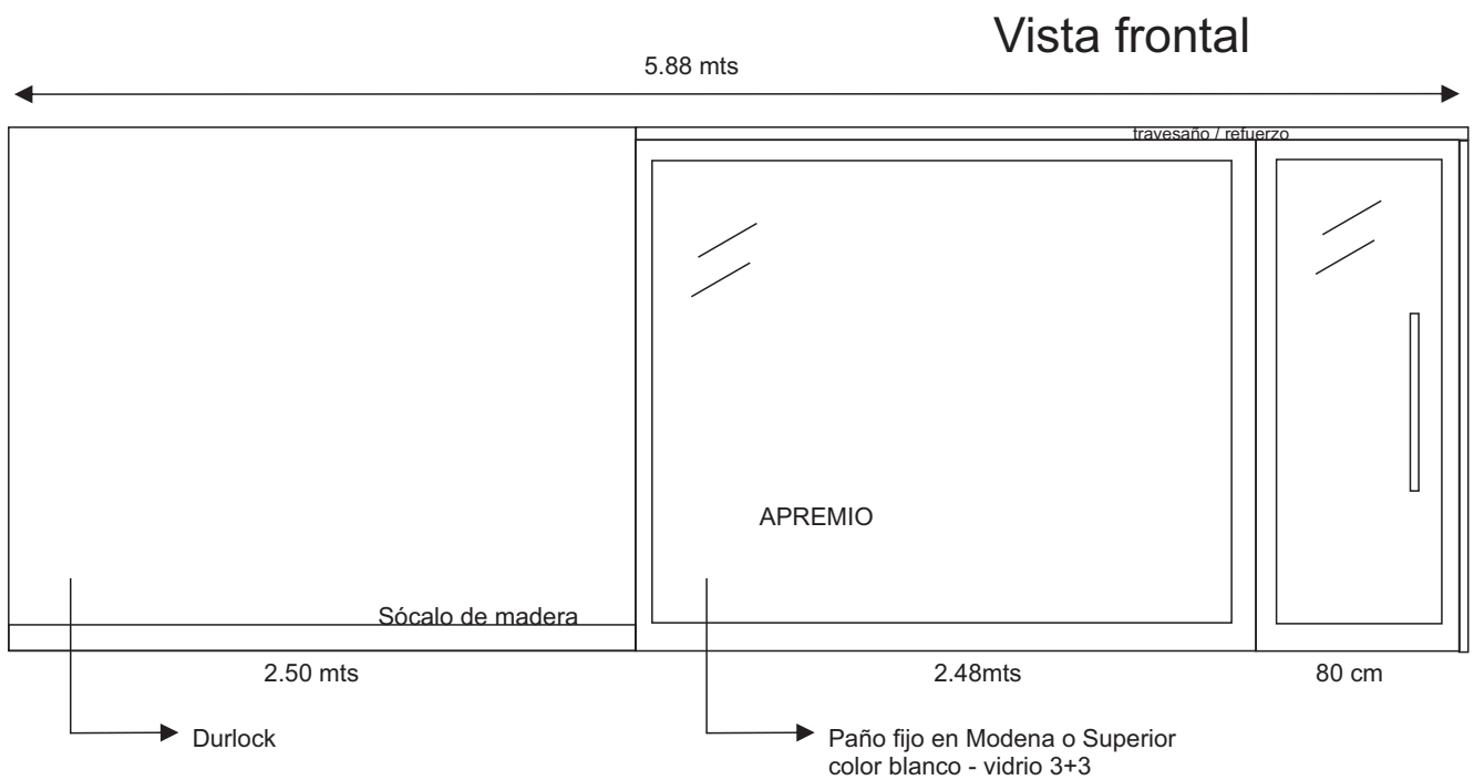
Fig. 2 - DIVISORIO DE DURLOCK y ALUMINIO (PERPENDICULAR A DIVISORIO DE DURLOCK)
