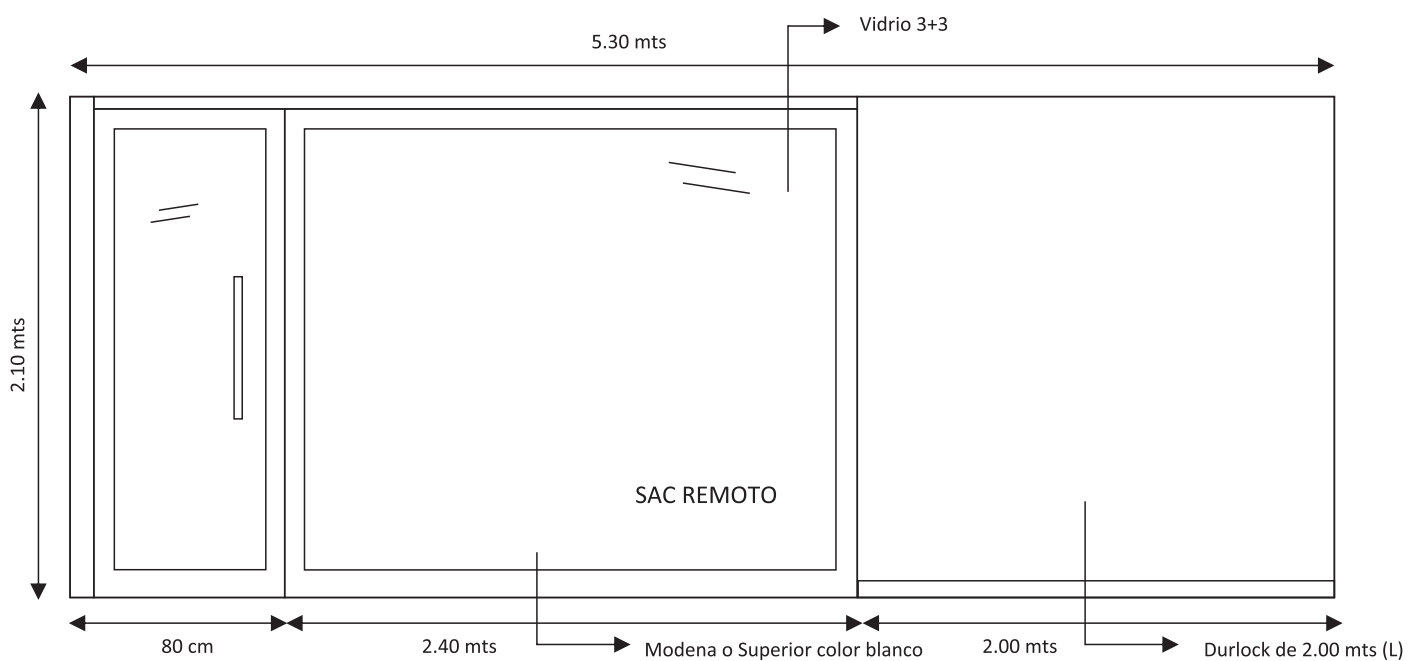
Fig. 4 - DIVISORIO DE DURLOCK (PERPENDICULAR A DIVISORIO DE DURLOCK)
