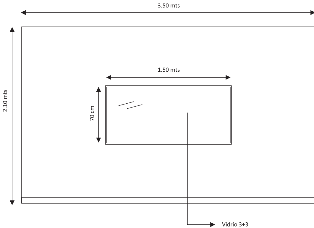
Fig. 4 - DIVISORIO DE DURLOCK (PERPENDICULAR A DIVISORIO DE DURLOCK)
