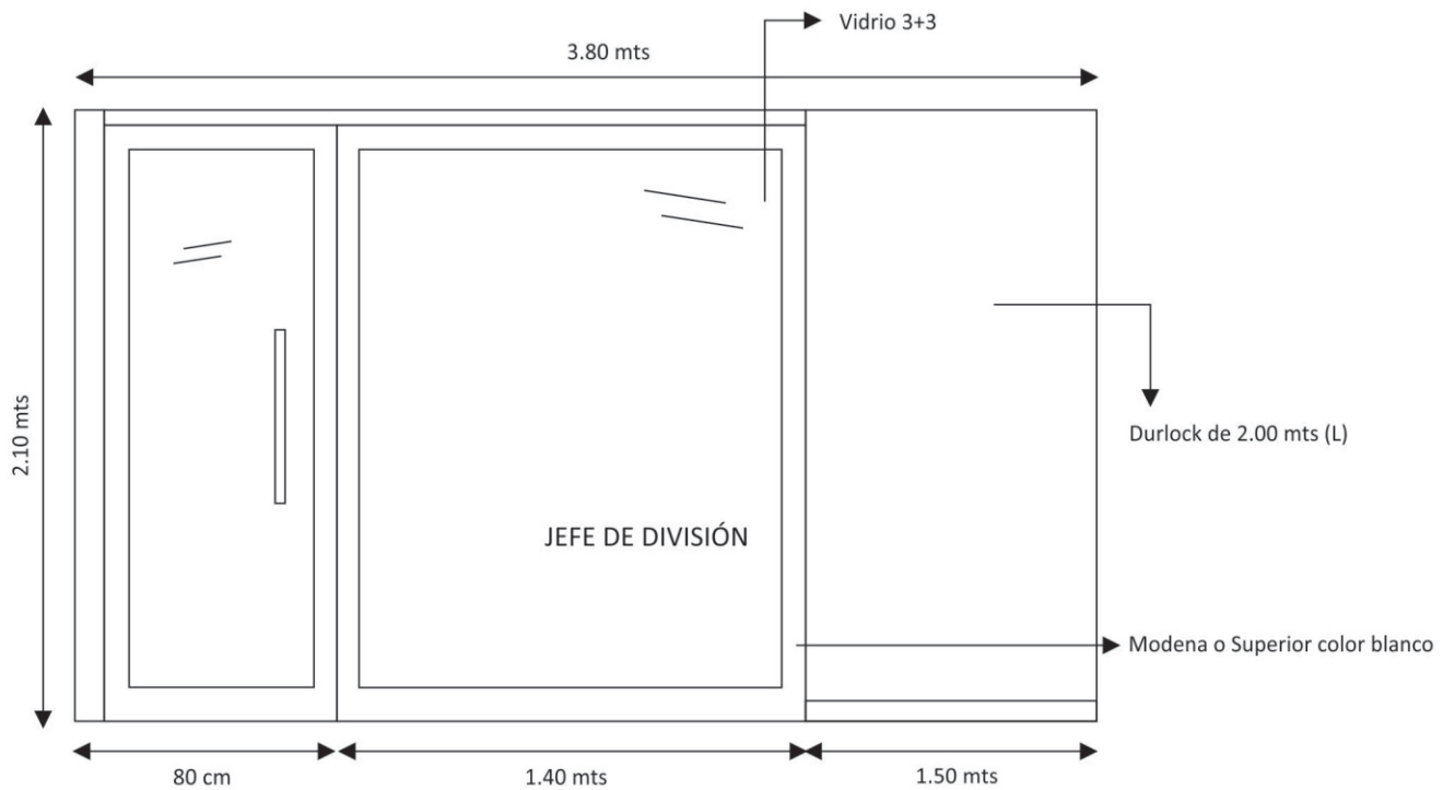
Fig. 2 - DIVISORIO DE DURLOCK (PERPENDICULAR A DIVISORIO DE DURLOCK)
