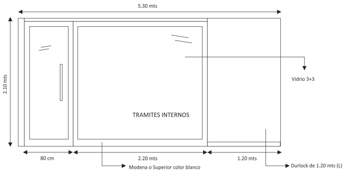
Fig. 2 - DIVISORIO DE DURLOCK (PERPENDICULAR A DIVISORIO DE DURLOCK)
