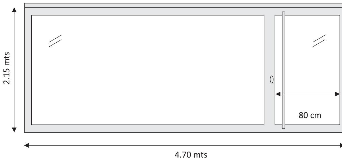
Fig. 2 - ESTRUCTURA DE ALUMINIO Y VIDRIO | REF. RESPONSABLE DE OFICINA
